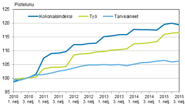
Kuvio 2. Kiinteistön ylläpidon kustannusindeksi 2010=100
