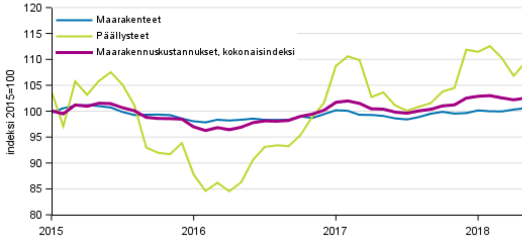
Liitekuvio 1. Maarakennusindeksin 2015=100 kokonaisindeksin, maarakennetöiden ja päällysteiden kustannuskehitys 1/2015–5/2018
