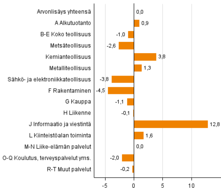
Kuvio 2. Toimialojen arvonlisäyksen volyymin muutokset 1. neljänneksellä 2015 vuodentakaisesta (työpäiväkorjattuna, prosenttia)
