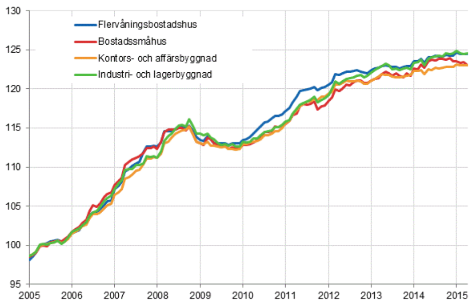
Figurbilaga 1. Byggnadskostnadsindex 2005=100
